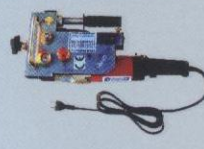
عملگر برقی سیار Torque: 0-450 N.m Source: 220 VAC 1 Phase 50 Hz
